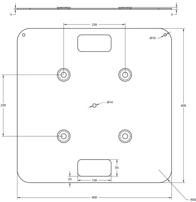
Embase inférieure
