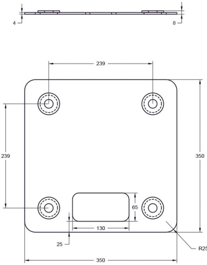
Embase supérieure
