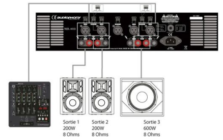
Utilisation du WA-4x3 en diffusion triphonique : Les enceintes larges bandes et le caisson de basse sont alimentés par le même amplificateur. Les réglages en façade permettent une optimisation de la diffusion.
